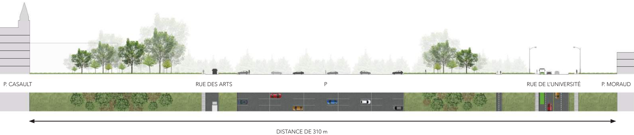
COUPE B
